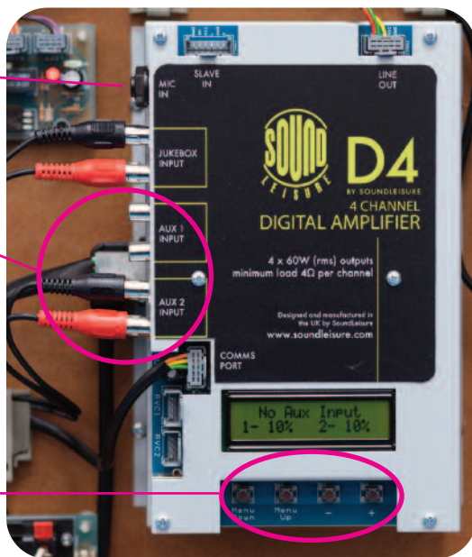
FIG 8 VUE DE L'AMPLIFICATEUR NUMÉRIQUE D4
